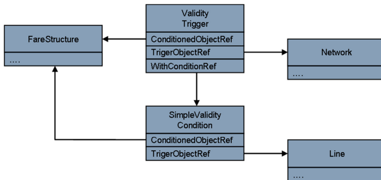
Figuur 21 Informatiemodel geANDde geldigheidconditie
