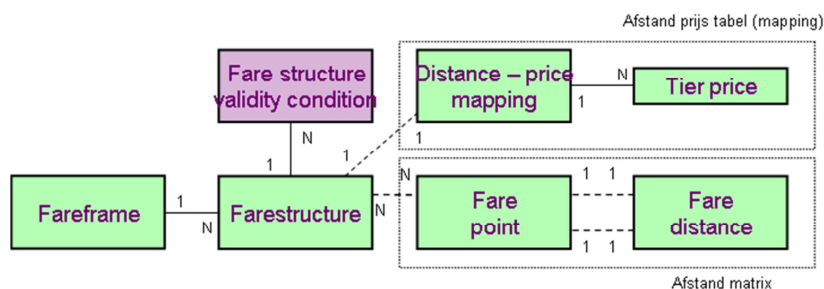
Figuur 8 Informatiemodel Staffeltabel
