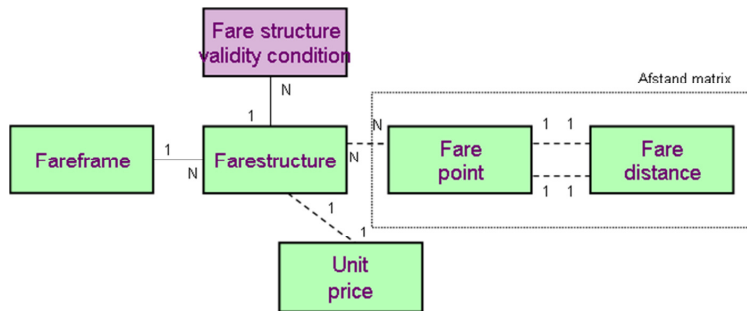
Figuur 7 Informatiemodel Eenheidsprijs
