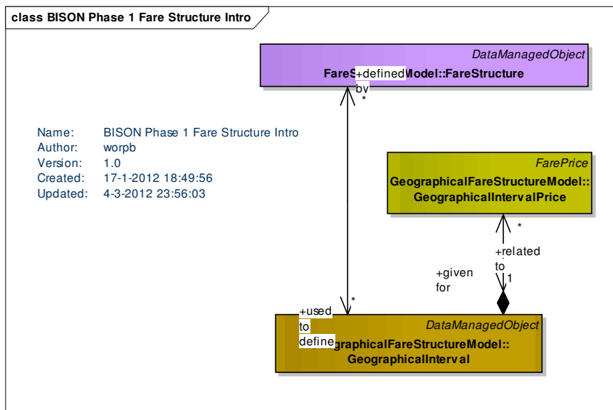
Figuur 19 UML, fysiek, fare structure met staffeltabel
