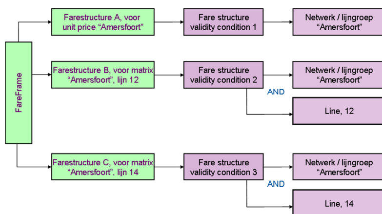
Figuur 12 Informatiemodel Voorbeeld eenheidsprijs
